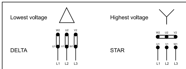
Image 6 Schéma de câblage d'un entraînement constant \Delta/Y 220/380V.
