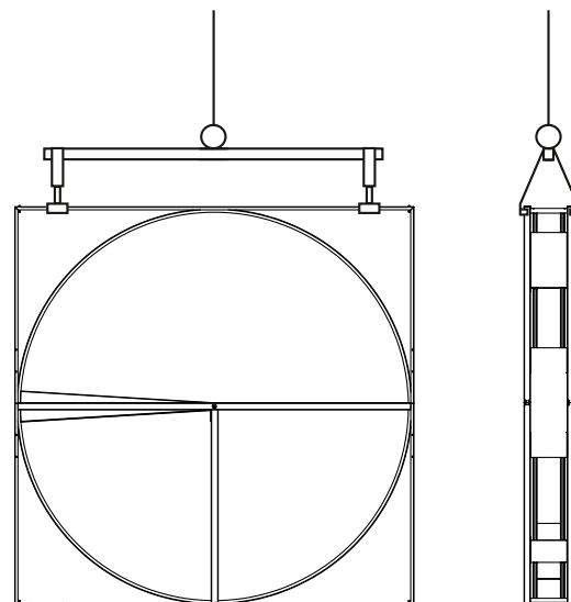
Image 2 Si le carter est couvert, soulevez le carter au niveau des bâtis.
