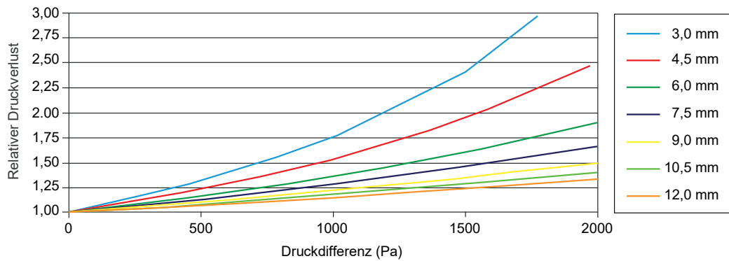
Abbildung 1. Auswirkungen der Druckdifferenz auf den Druckverlust, Modell H.
