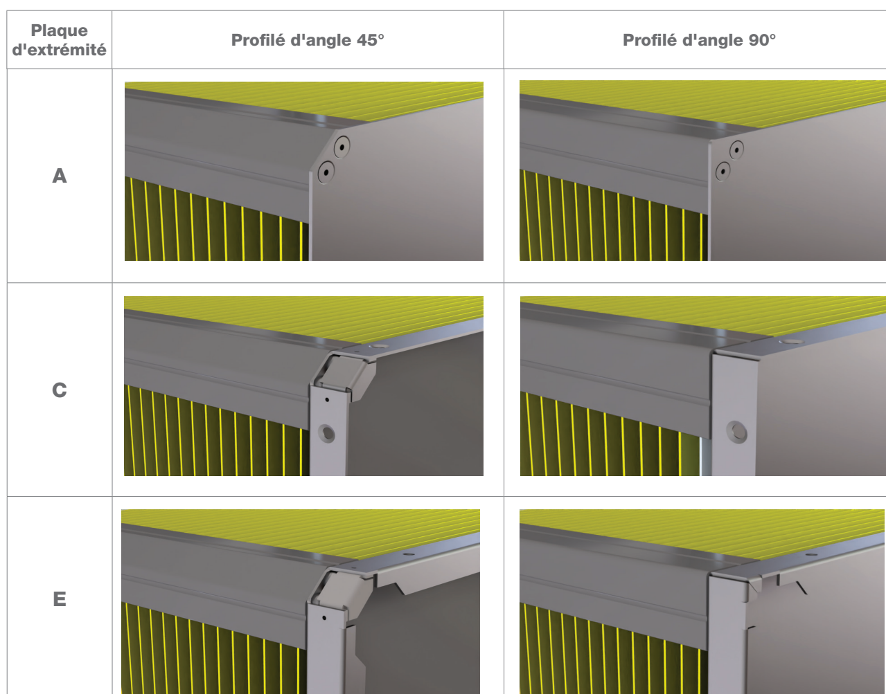
Image 10. Plaques d'extrémité et profilés d'angle
